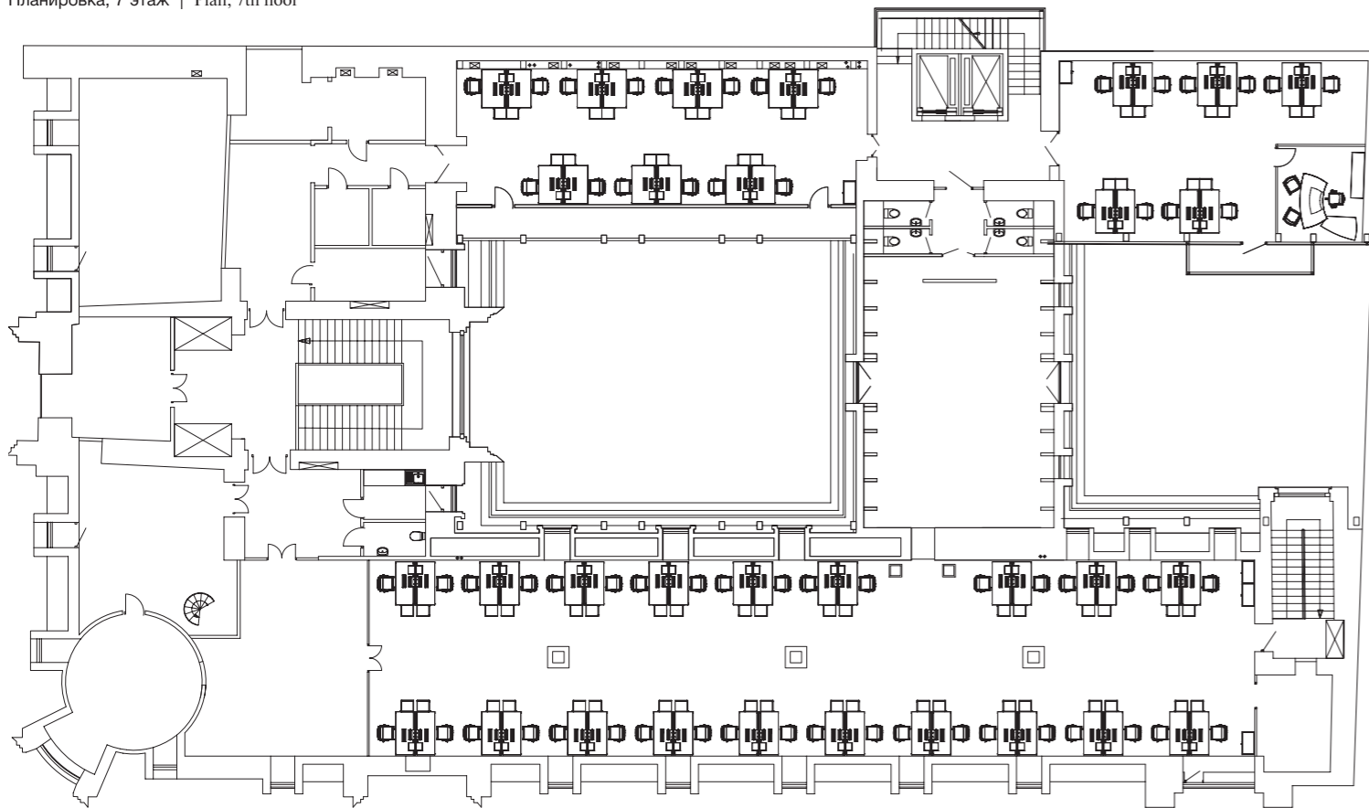
Планировка, 7 этаж | Plan, 7th floor
